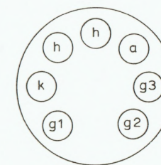
CV138 EF91
