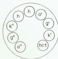
CV492 12AX7
