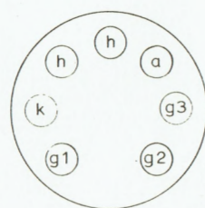
CV131 EF92
