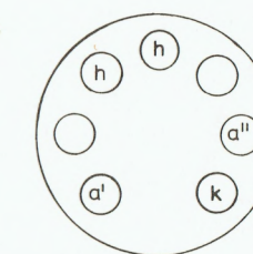
CV493 or CV4005 6X4
