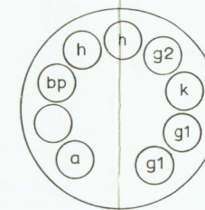
CV2129 or CV4039 5763
