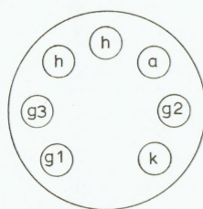
CV454 or CV4009 6BA6
