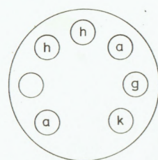
CV133 or CV4058 6C4
