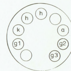
CV2127 or CV4055 6CH6
